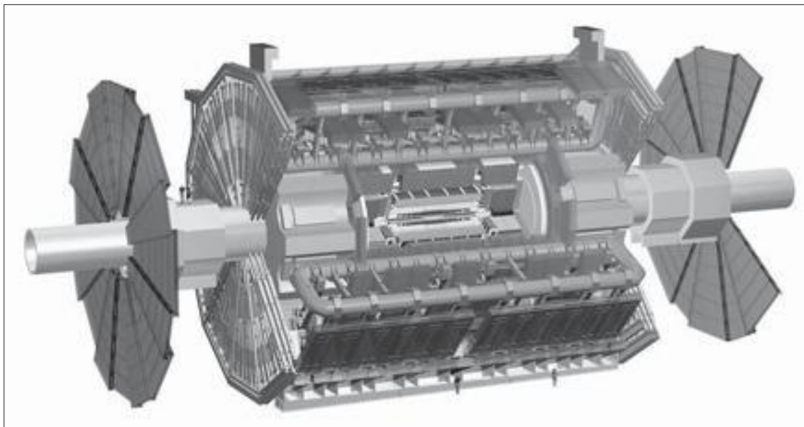
Ryc. 12.84. Schemat detektora ATLAS
