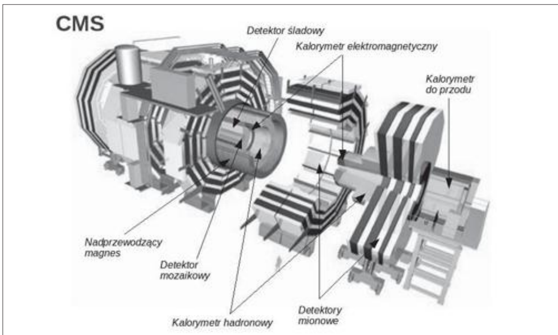
Ryc. 12.85. Schemat detektora CMS
